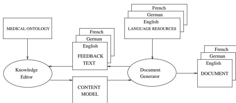
Figure 2: WYSIWYM editing
